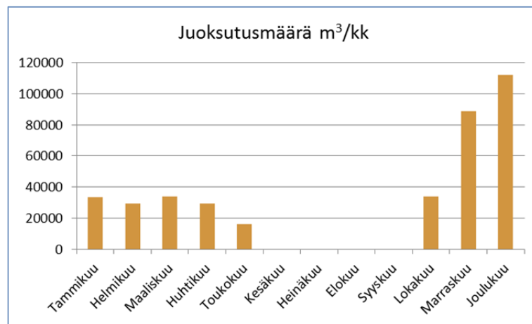
Kuva 7.2. Vihtilammista Säcksjärveen juokutettu vesimäärä, m 3 /d, kuukausittain vuonna 2017.
