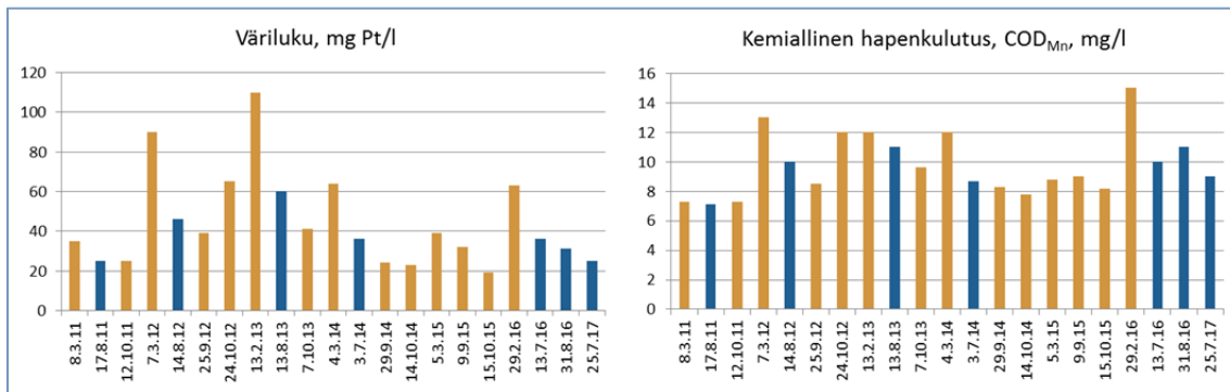
Kuva 5.1. Veden humustilaa kuvaavat väriluvun ja kemiallisen hapenkulutuksen arvot Vihtilammissa vuosina 2011-2017. Kuvassa heinä-elokuun arvot ovat sinisiä pylväitä.
