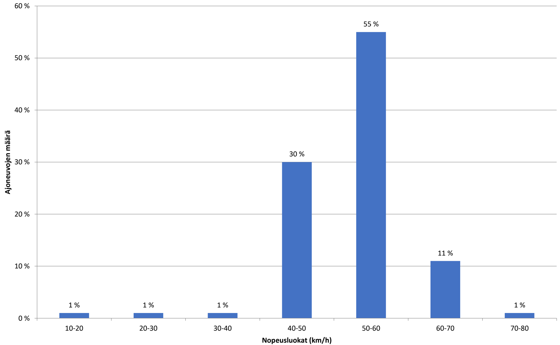
Nopeusjakauma - Koko mittaus - Piste 2 Suunta 2
