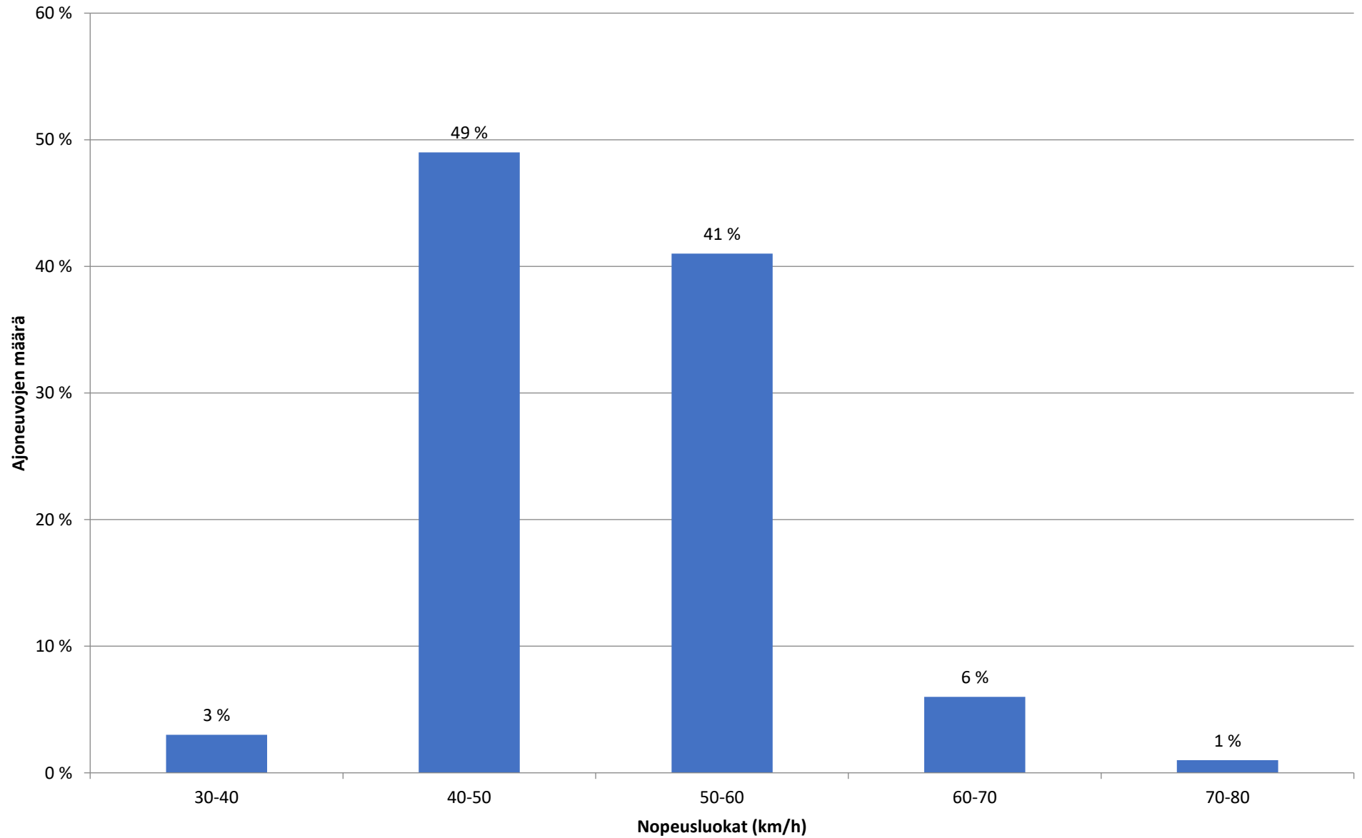
Nopeusjakauma - Koko mittaus - Piste 2 Suunta 1
