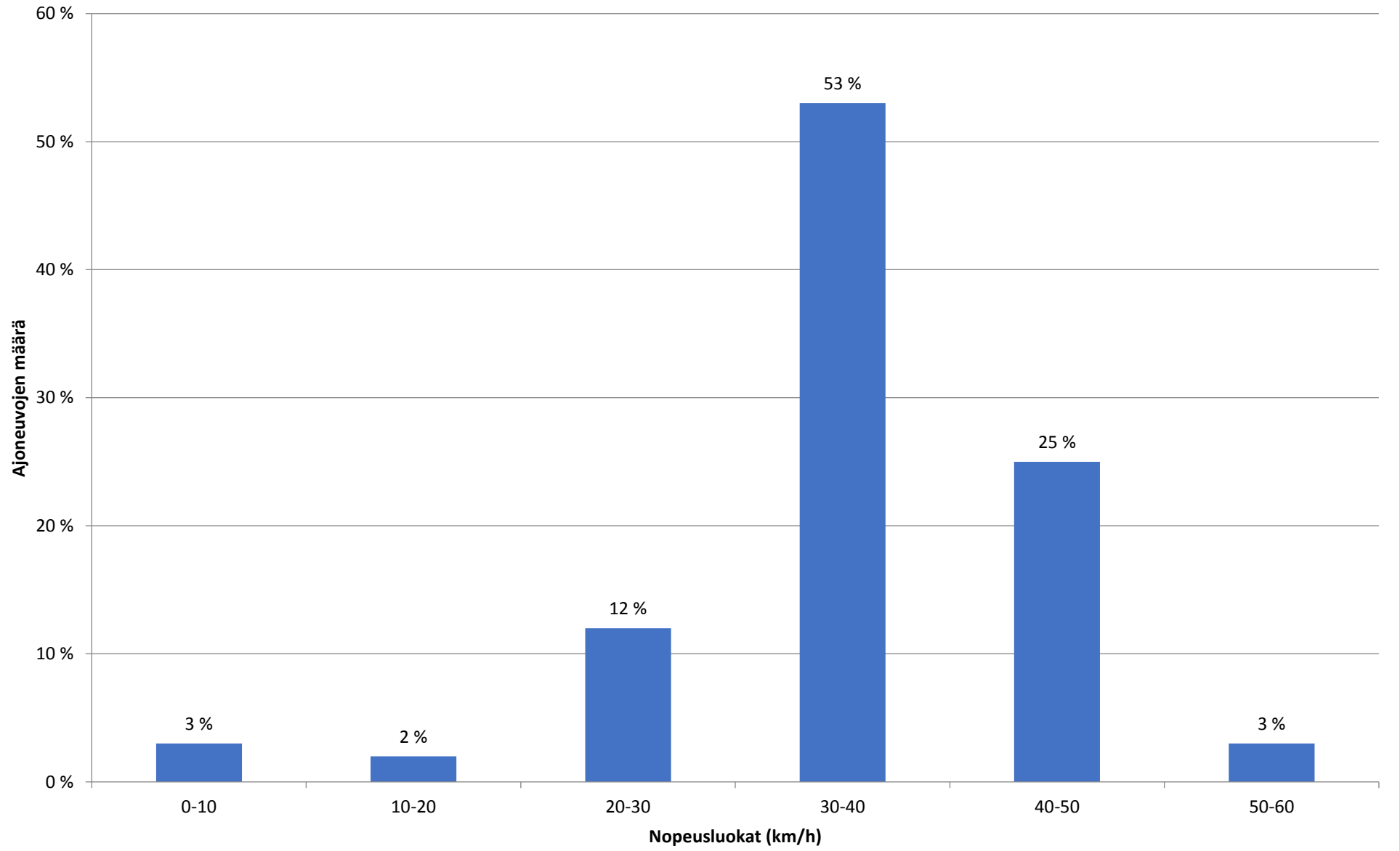
Nopeusjakauma - Koko mittaus - Piste 4 Suunta 1
