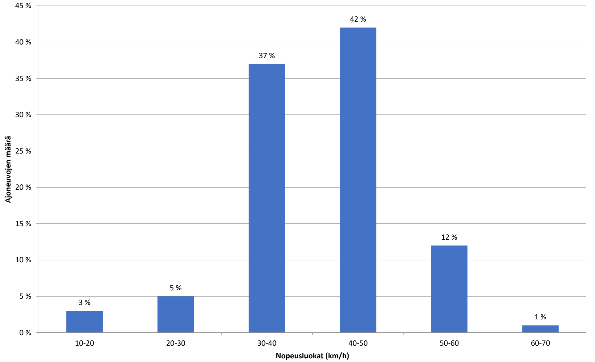
Nopeusjakauma - Koko mittaus - Piste 5 Suunta 2
