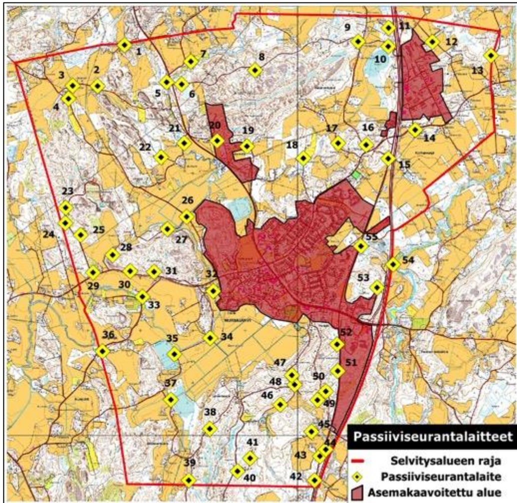
Kartta 3. Passiiviseurantalaitteiden sijainnit selvitysalueella 2013.
