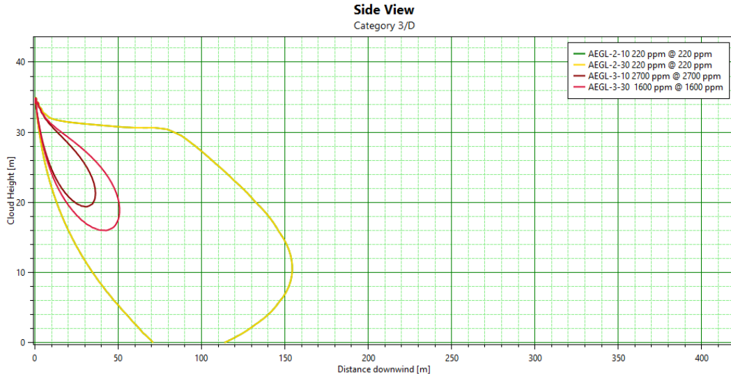
Kuva 5. Sivuleikkauskuva ammoniakkivuodon leviämisestä ympäristöön, kun ulospurkausputkesta vuoto suuntautuu alaspäin 45 asteen kulmassa ja vuotokorkeus on 35 metriä. Punainen väri kuvaa AEGL-3-10, tummanpunainen on AEGL-3-30 ja keltainen on AEGL-2-30.
