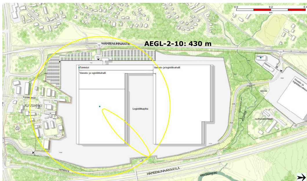
Kuva 12. Ammoniakkipäästön AEGL-2-10 (220 ppm) vaikutukset esitettynä kartalla 25 metrin vuotokorkeudesta suuntautuen alaspäin 45 asteen kulmassa varoventtiilin sijaitessa logistiikkakeskuksen eteläisen osan keskellä.
