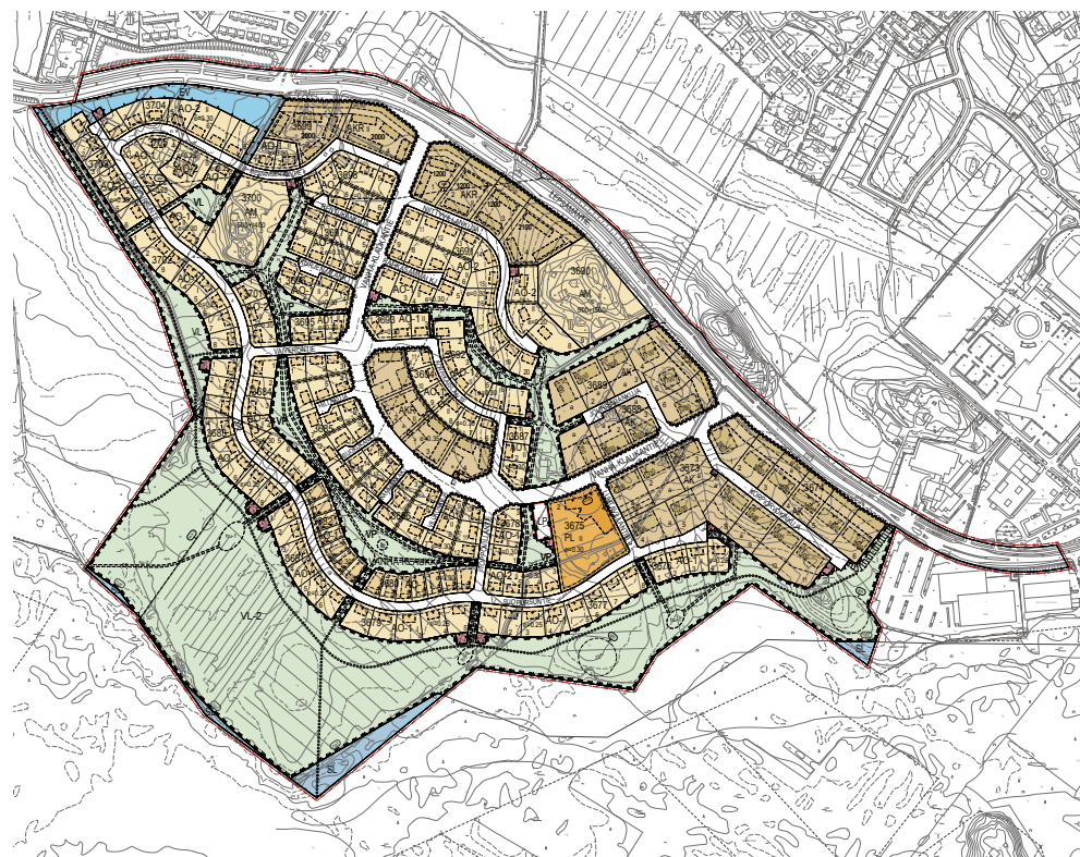
Kuva 2. Vanha-Klaukan asemakaava.
