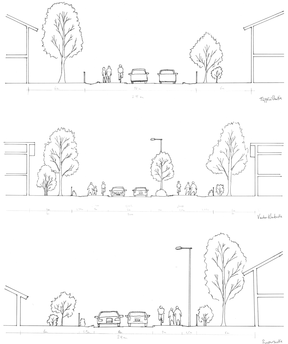
Kuvat 14 (ylin), 15 ja 16 (alin). Katujen luonteita ja tilallisuutta on tutkittu kavasuunnittelun yhteydessä poikkileikkauksin.
